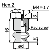
VP10, 15B 5 -M4
