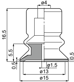
VP15B [5]- Q [8] Weight : 1.8g[2.5g]
